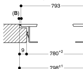
Przekrój podłużny
